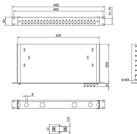
D. Dimensions du produit (vues avant, de dessus et arrière) et des bras de fixation en mm
